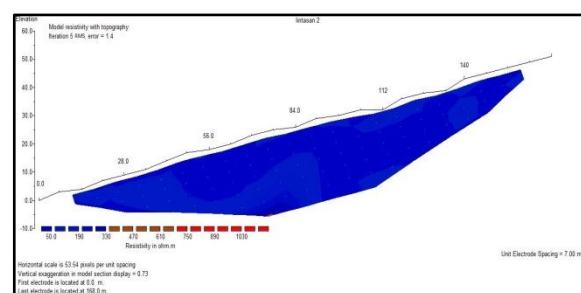
Gambar 4 Pemodelan 2D Lintasan-2 dengan efek topografi
