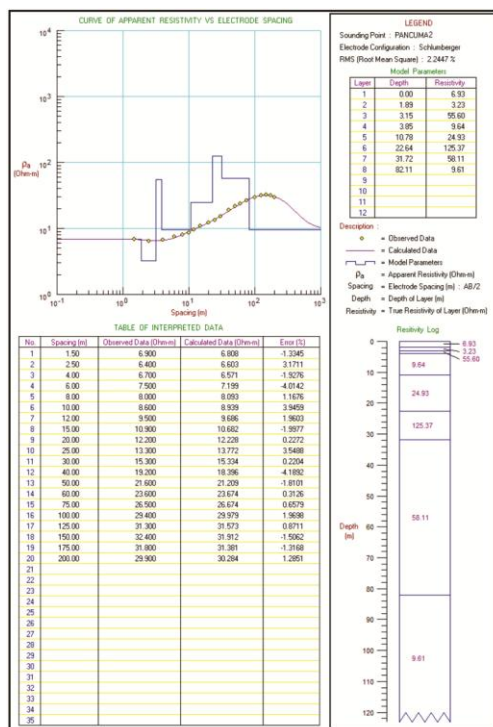
Gambar 7. Hasil Pengolahan VES Titik Duga 2
