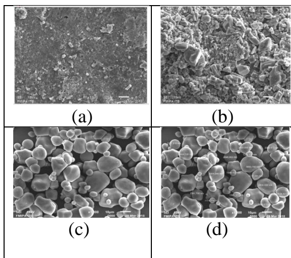
Gambar 2. Morfologi (a) karaginan kasar, (b) karaginan kasar-ekstrak etanol, (c) karaginan murni-ekstrak etanol, (d) karaginan murni-ekstrak etanol.
